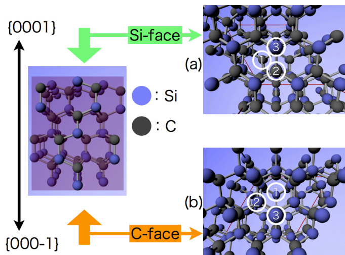
図 21: 4H-SiC の (a) Si-face (b) C-face における C 原子の吸着位置.
