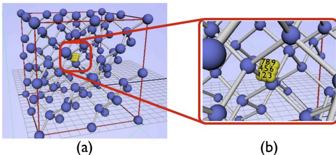
図 12: Si 完全結晶内に O 原子を配置した構造モデル。 (a) Si スーパーセル, (b) O 原子の配置面。
