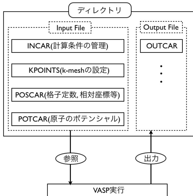
図 34: VASP の計算のプロセス. ディレクトリの中に 4 つの入力ファイルを用意して VASP を実行. 計算終了後, 結果をディレクトリに出力する.
