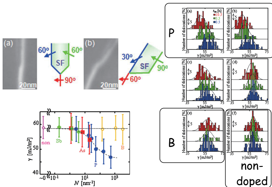
図 26: 模式図で示したような転位の分解挙動の weak beam 法による電子顕微鏡鏡像、この幅を測定し集計したヒストグラム、および、それから求めた stacking fault energy の dopant 濃度依存性。
