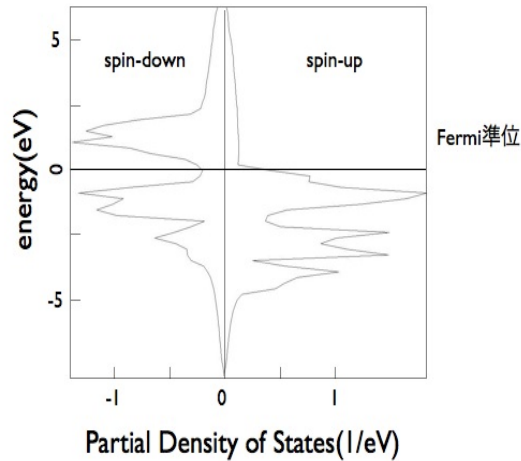
図 51: 強磁性を示す bcc-Fe の上向きスピン (spin-up) と下向きスピン (spin-down) の状態密度図。
