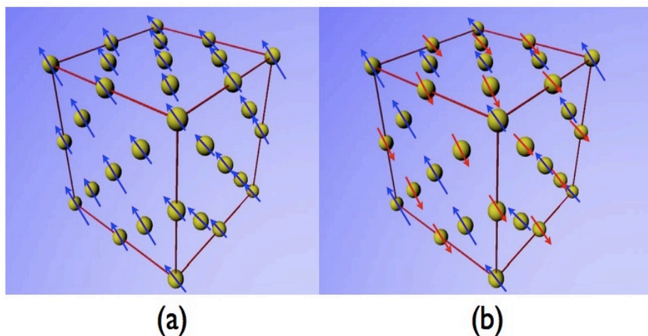
図 52: (a) 強磁性体, (b) 反強磁性体のモデル。
