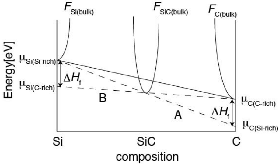
図 24: Si-C の系の組成・自由エネルギー図。横軸において、左端が Si100 %，右端が C100 %を示し，SiC は組成比 1:1 なので，中心に位置する。縦軸はエネルギーを示す。
