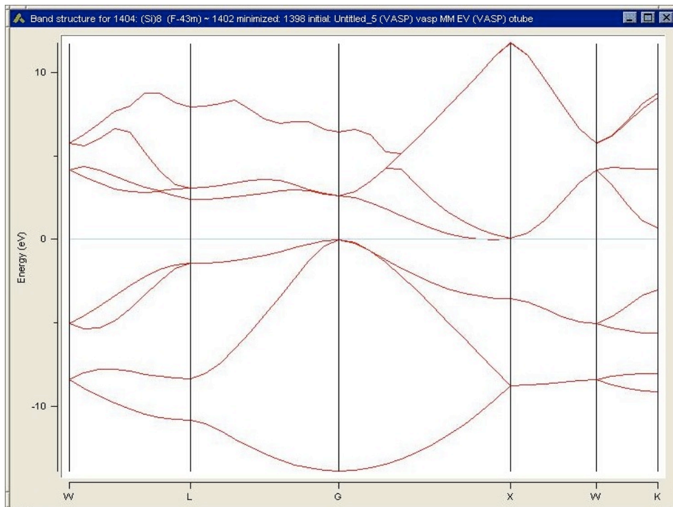
図 50: Si のバンド構造.
