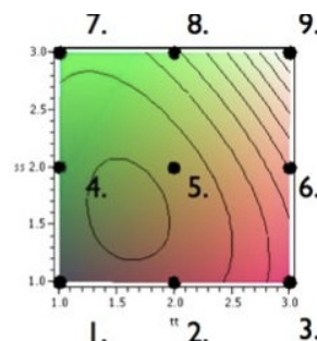
図 5: Si 原子のボンドの中間位置に酸素原子を 図 6: 左のモデルの各点に対応する断熱ポテンシャル面, 9 カ所指定して挿入した模式図.
