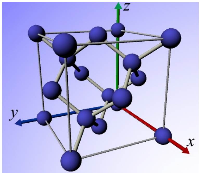
図 39: Si のダイヤモンド構造
