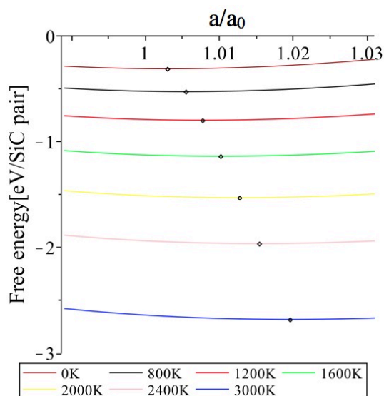
図 17: 各温度における 3C-SiC の自由エネルギーの格子定数依存性。
