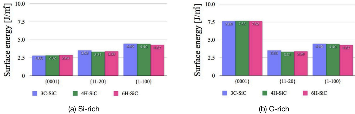
図 25: SiC の多形ごと, 表面ごとの表面エネルギー.
