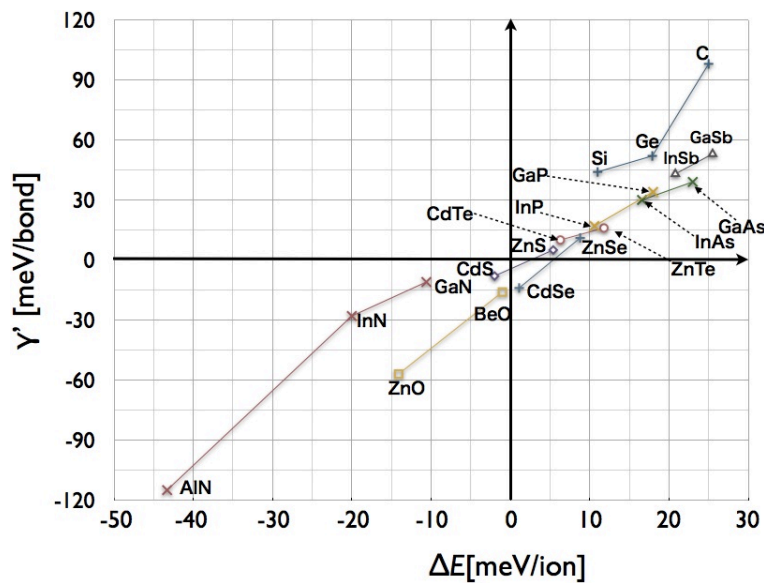
図 8: 積層欠陥エネルギー ( \gamma' ) と, ZB と WZ の構造エネルギー差 ( \Delta E_{ZB-WZ} ) との相関.
