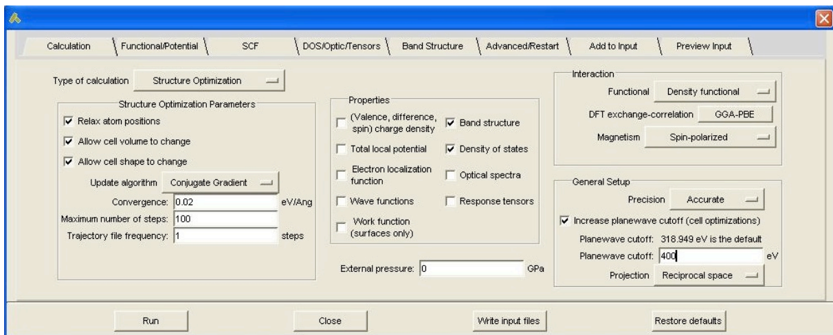
図 47: 計算に必要なパラメータの設定 (構造緩和, DOS やバンド構造出力等の設定)。
