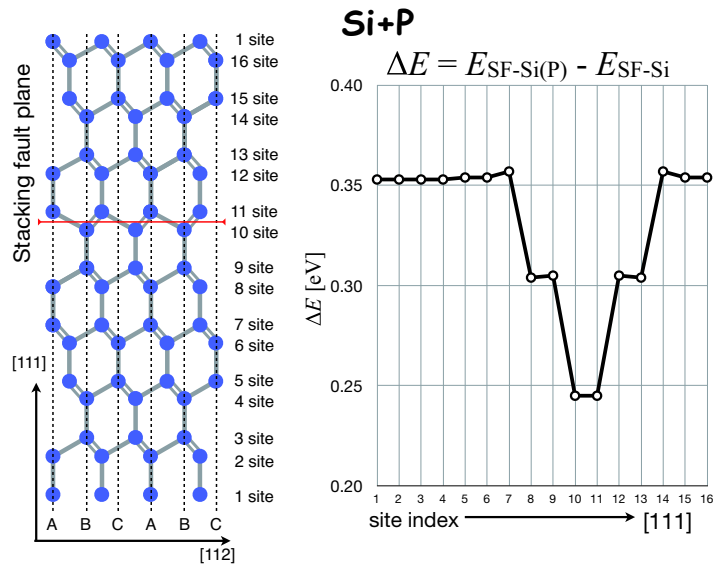
図 27: 原子配置の模式図と、それぞれの層の Si 一原子を P と置換した場合のエネルギー変化.
