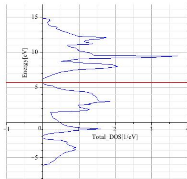
図 45: diamond 構造の Si の電子状態密度分布 (electron DOS:electron density of states). 縦軸が Energy[eV], 横軸が DOS[1/eV] (状態密度) である.
