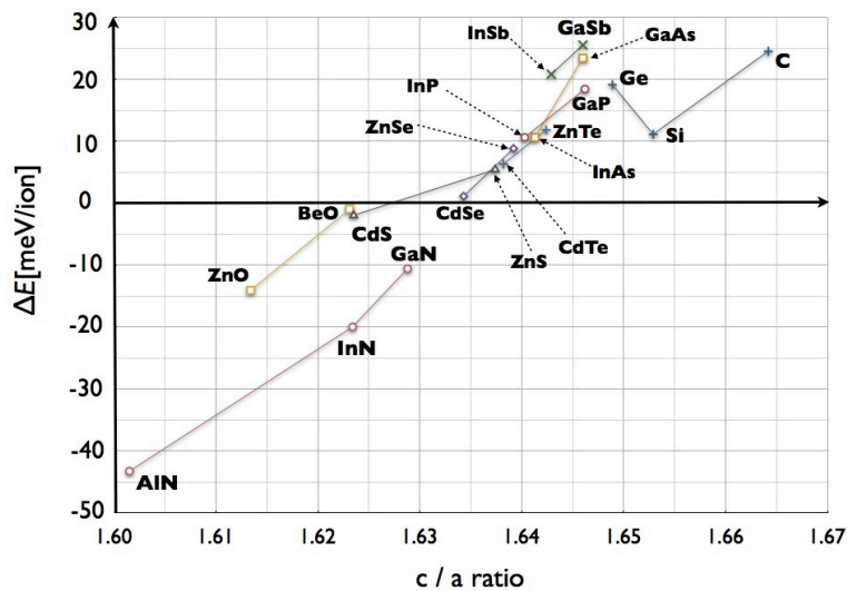
図 9: 構造エネルギー差 ( \Delta E_{ZB-WZ} ) と, WZ の c/a 比 との相関.
