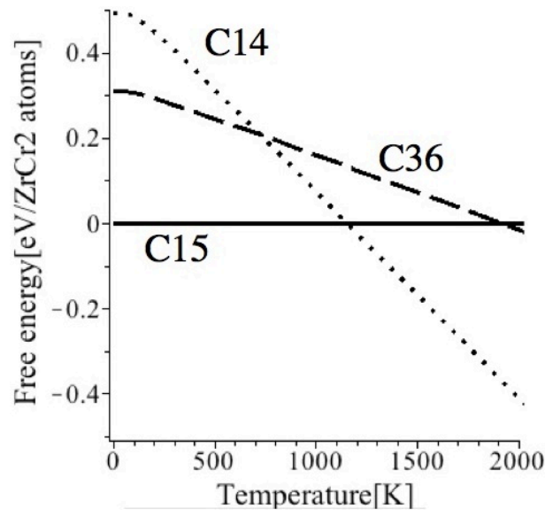
図 16: ZrCr 2 Laves 相における結晶多形の自由エネルギーの温度依存性。
