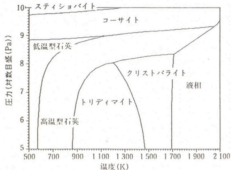
図 10: SiO 2 多形の状態図。
