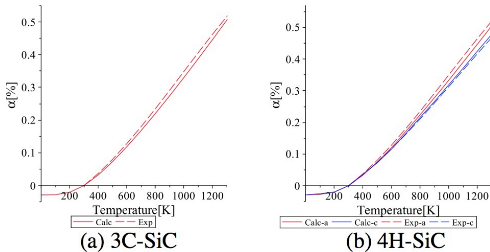
図 19: (a)3C-SiC (b) 4H-SiC における線形膨張率の温度依存性.
