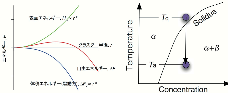
図 29: 核生成にともなう自由エネルギー変化のクラスター半径依存性。固体の析出現象の状態図による解説。
