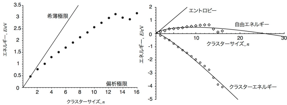
図 32: 偏析極限からの差で示した最安定エネルギーのクラスターサイズ依存. Cu のクラスターサイズによる自由エネルギー変化. エントロピーは焼鈍温度 773K, 初期組成 1.4%Cu として求め, 曲線は計算値にフィットしてある.
