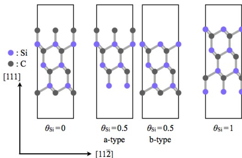
図 23: 表面を覆う Si 原子の割合を \theta_{\text{Si}} とし、Si-rich, C-rich の環境を考慮したスラブモデルの模式図。なお \theta_{\text{Si}} = 0.5 の場合、図のように a-type と b-type のモデルを作成した。
