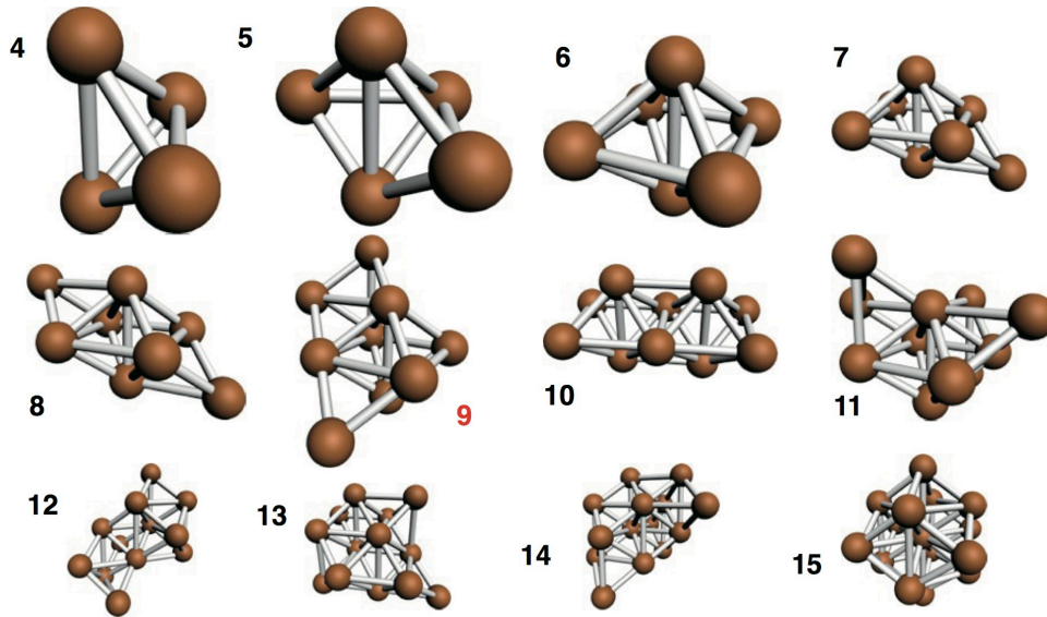
図 31: クラスターサイズ n で最安定エネルギーを示した原子の配置.
