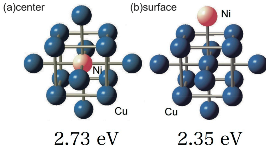
図 33: 第 3 元素として Ni を添加した場合の中心と表面のモデル.
