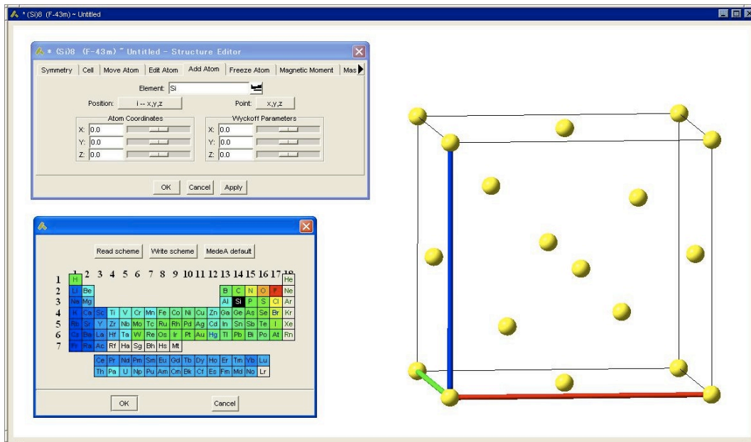
図 46: 計算に必要なパラメータの設定 (構造緩和, DOS やバンド構造出力等の設定)。
