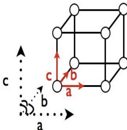
図 4: 格子構造のモデル. 実線の矢印が内部緩和に関する軸を, 点線の矢印が外部緩和に関する軸ベクトルをあらわす.
