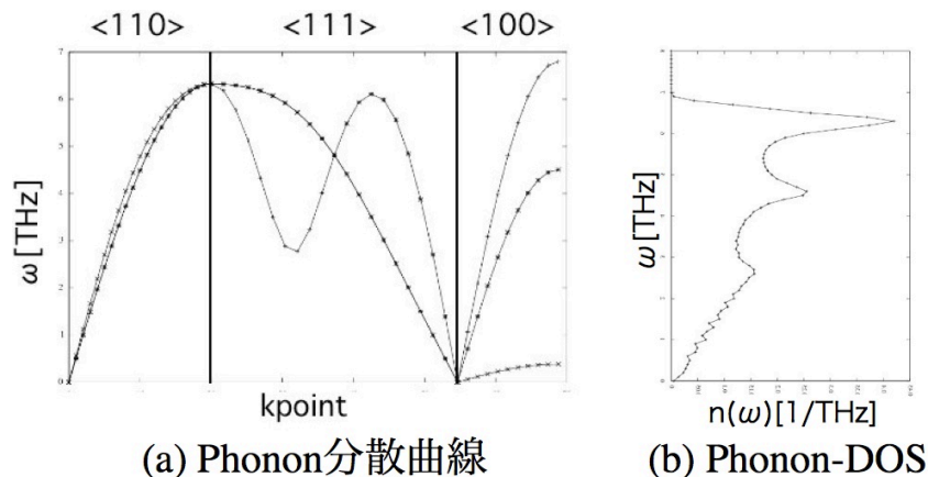
図 55: アルミニウムにおける (a) Phonon 分散曲線, (b) Phonon-DOS.
