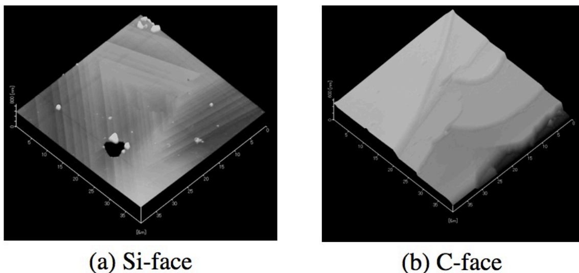
図 20: 4H-SiC の (a) Si-face および (b) C-face の走査トンネル顕微鏡像。
