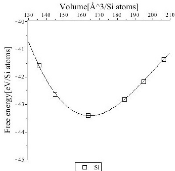
図 3: Si の E-V 曲線 (energy-volume curve, エネルギー体積曲線).
