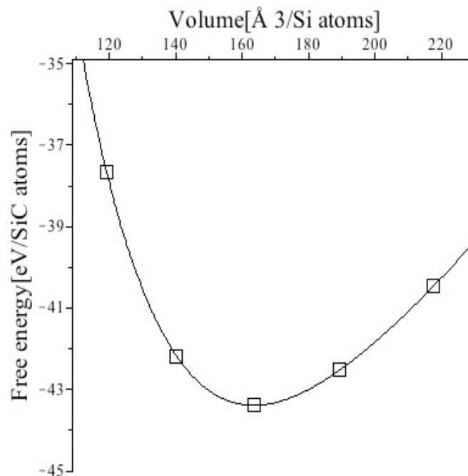
図 36: Si の E-V 曲線
