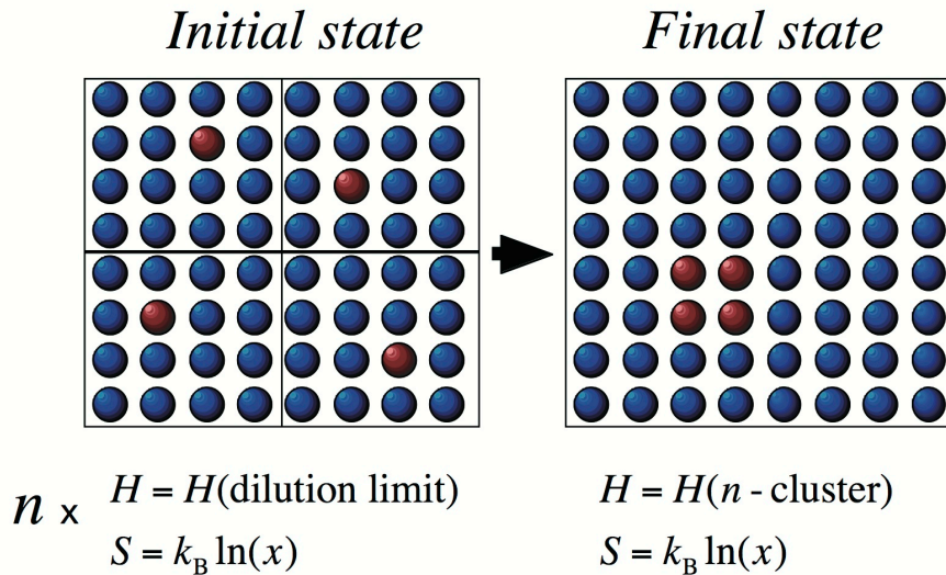
図 30: 析出核の自由エネルギー変化の始状態と終状態を示すモデル。
