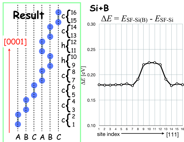
図 28: 原子配置の模式図と、それぞれの層の Si 一原子を B と置換した場合のエネルギー変化.
