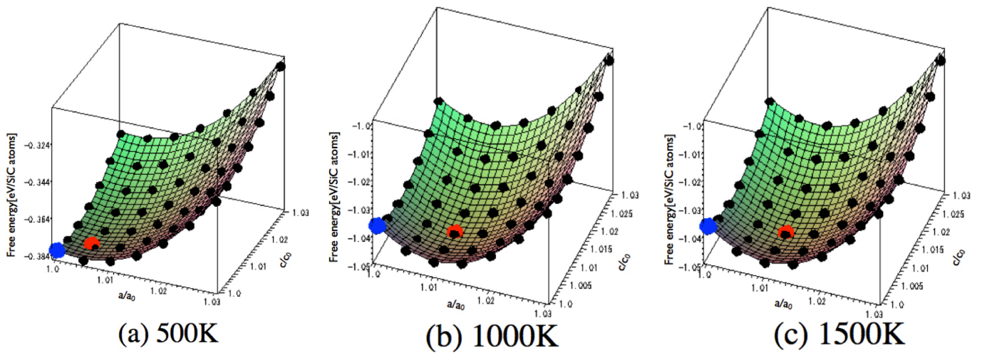
図 18: (a) 500K (b) 1000K (c)1500K における 4H-SiC の自由エネルギーの格子定数依存性.
