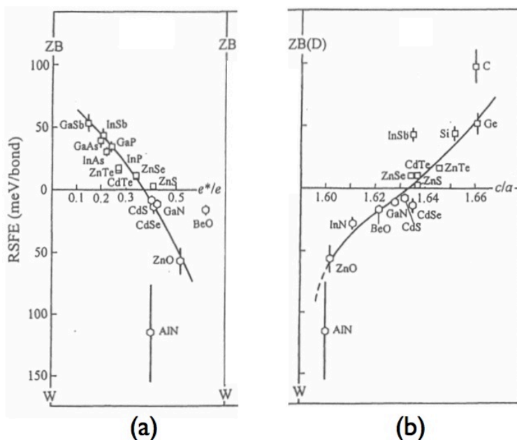
図7: 積層欠陥エネルギー ( \gamma' ) との相関. (a) 有効電荷 e^* , (b) WZ 構造の c/a 比.
