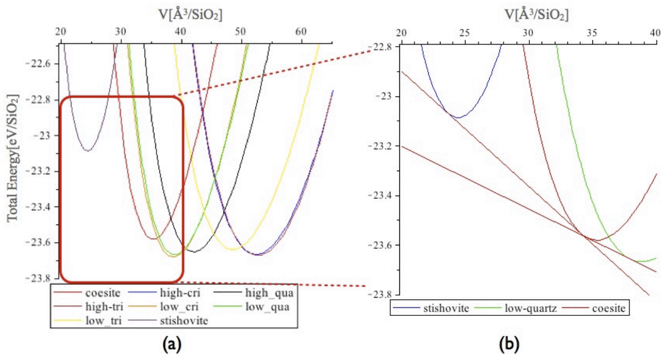
図 11: SiO 2 多形の E-V 曲線. (a) 多形 8 種の E-V 曲線. (b) stishovite と coesite, coesite と low quartz の共通接線.
