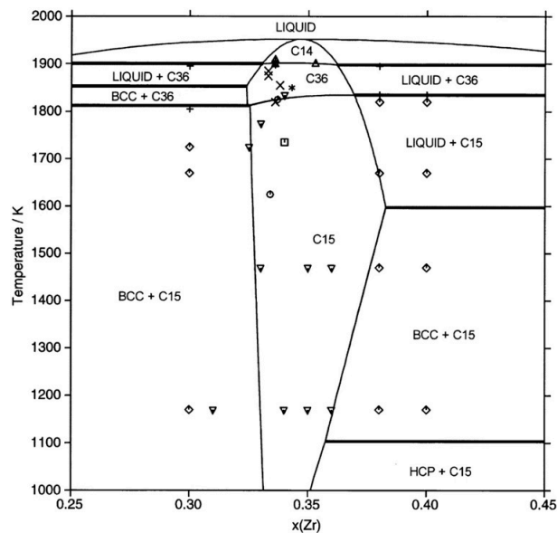
図 15: Zr-Cr 二元系状態図.
