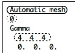
図 41: Siのダイヤモンド構造のKPOINTS ファイル。
