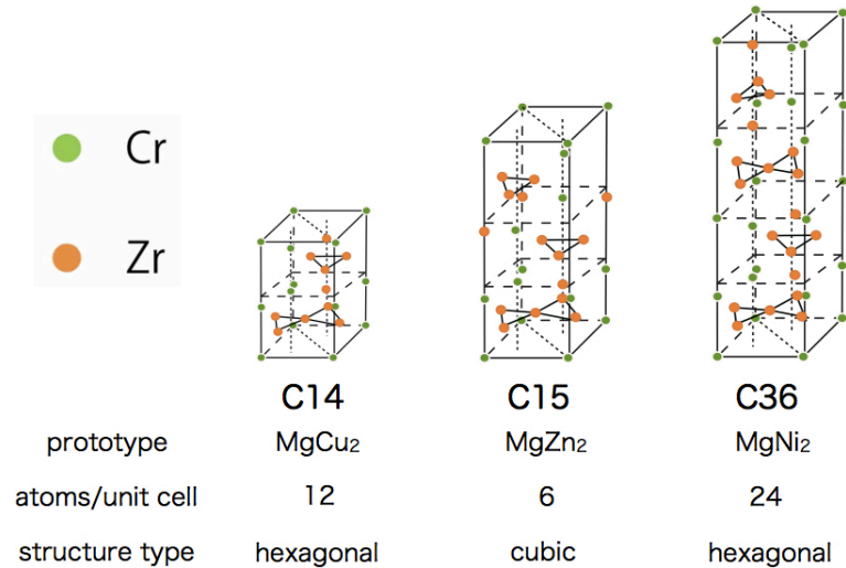
図 14: ZrCr 2 Laves 相の各積層構造.
