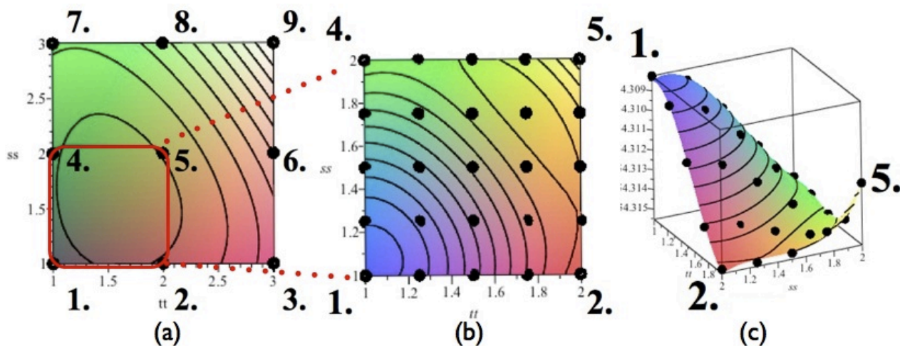
図 13: O 原子の侵入位置の違いによるエネルギー曲面図. (a) 求めたエネルギー曲面. (b) site1, 2, 4, 5 で囲まれた範囲のエネルギー曲面図. (c) (b). を斜め上方からみたエネルギー曲面の 3 次元図.
