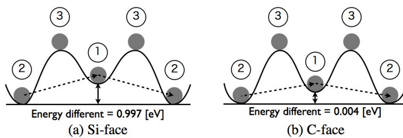
図 22: (a)Si-face (b)C-face での C 原子の活性化エネルギーの模式図.
