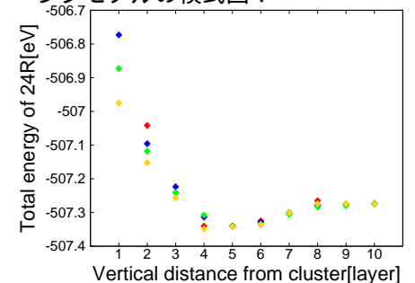
図 2 L_{12} クラスタと small cluster の距離によるエネルギー変化。グラフの点の色は図 1 で示した近接距離の色に対応している。
