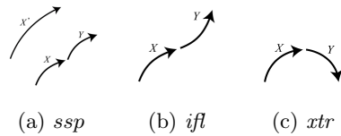
図 2 直接連結可能な単位セグメントのペア
