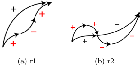
図 6 簡約規則と対応する図
