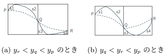
図 15 連結点の縦の位置関係
