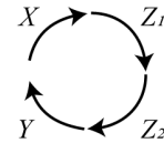
図5 閉埋め込みしか存在しない scurve
