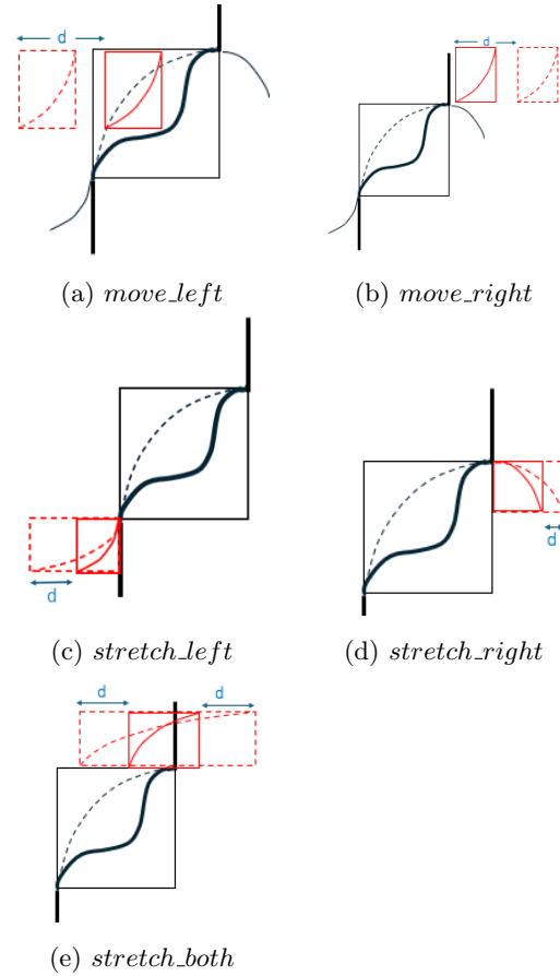
図 10 セグメント変形の操作 (r1)
