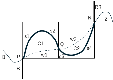
図 12 簡約規則 (r2) に関する表記 ( y_p < y_q < y_r のとき)
