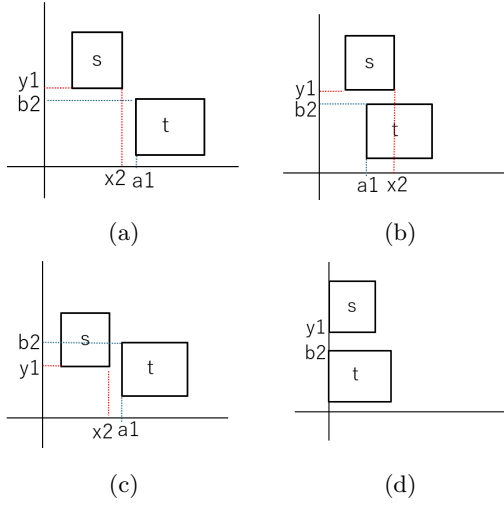
図 11 Right でのセグメント領域同士の位置関係 ( y_1 \leq b_1 のとき)
