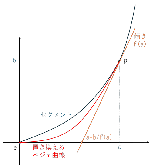
図 7 ゆるい連結からきつい連結への変換
