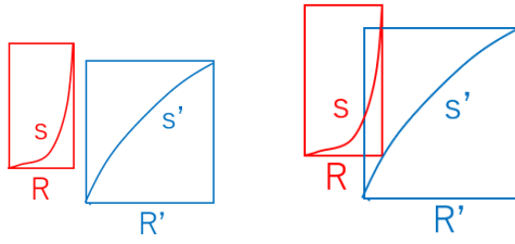
図 8 セグメント領域同士の位置関係
