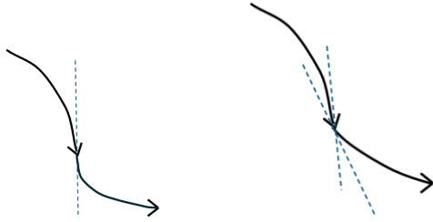
(a) きつい連結 (b) ゆるい連結
