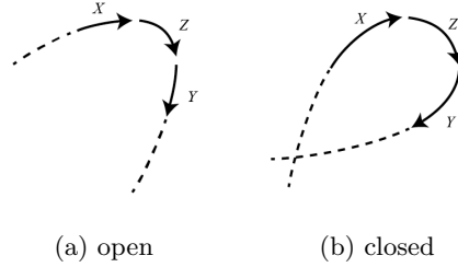
図4 X \cdot Z \cdot Y の 2 種類の埋め込み
