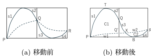
図 14 連結点の移動 ( y_p < y_r < y_q のとき)
