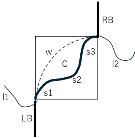
図 9 簡約規則 (r1) に関する表記
